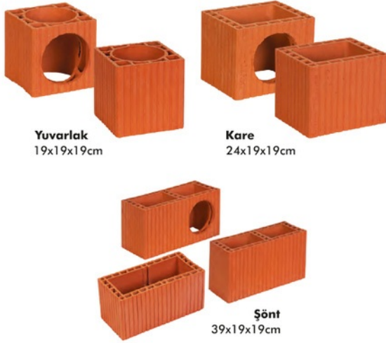
Normal Baca Uygulaması
